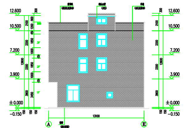
①-③轴立面图 1:100
