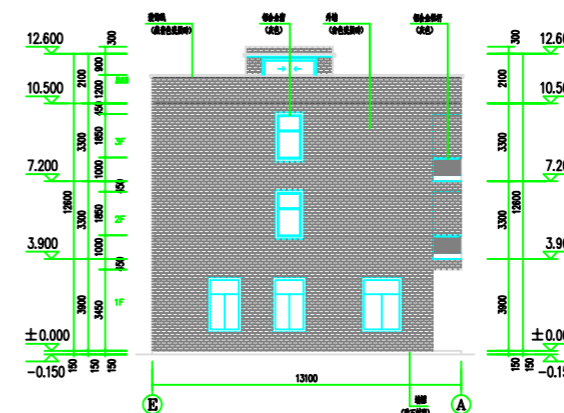
③-①轴立面图 1:100
