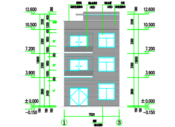
①-①轴立面图 1:100
