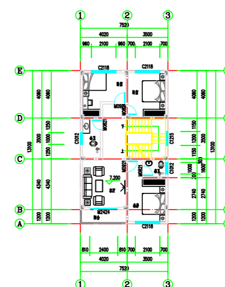
三层平面图 1:100
