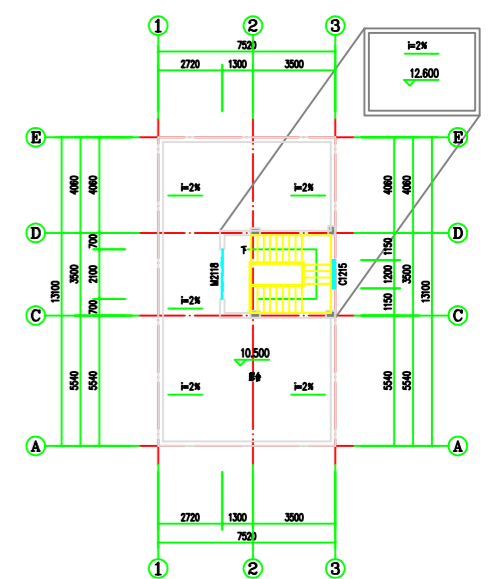
屋顶平面图 1:100
