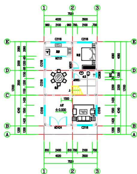
首层平面图 1:100
