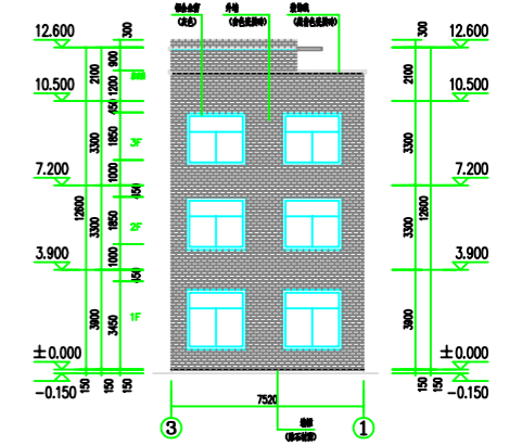
③-③轴立面图 1:100
