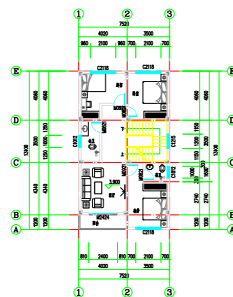
二层平面图 1:100
